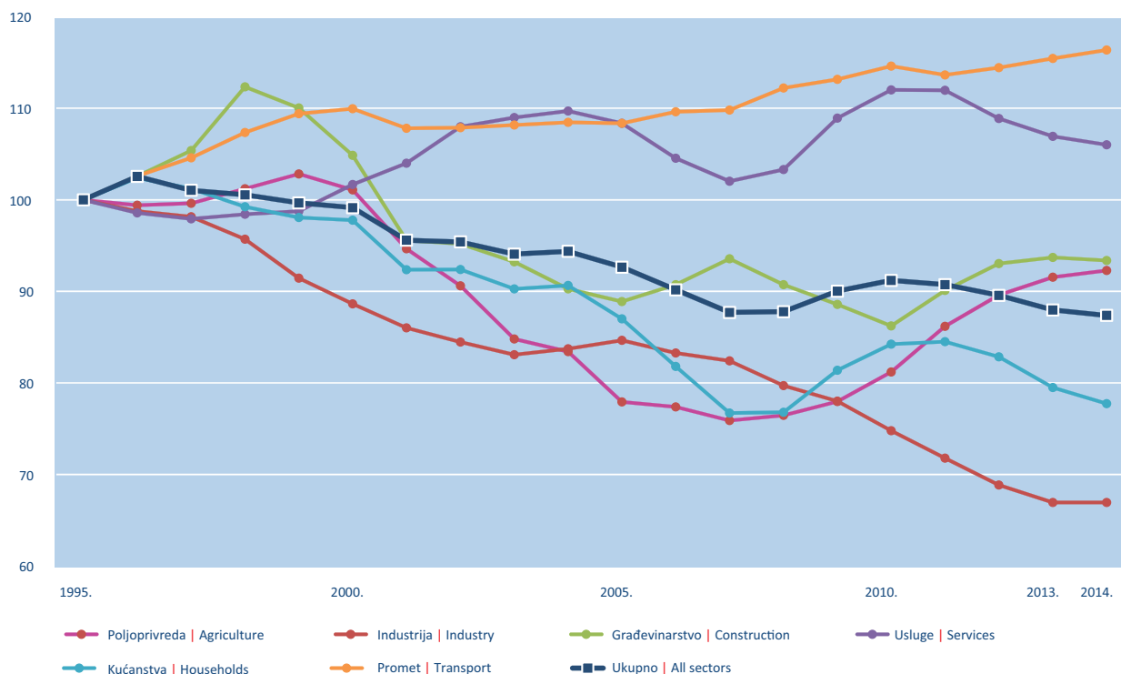
Slika | Figure 9.1.2. Indeksi energetske intenzivnosti u razdoblju od 1995. do 2014. godine | Energy intensity indices between 1995 and 2014 – Izvor | Source: EIHP
