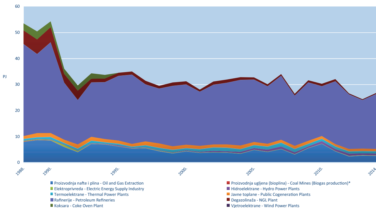
Slika | Figure 2.9.3. Pogonska potrošnja energije u energetske postrojenjima | Energy sector own use by plants
