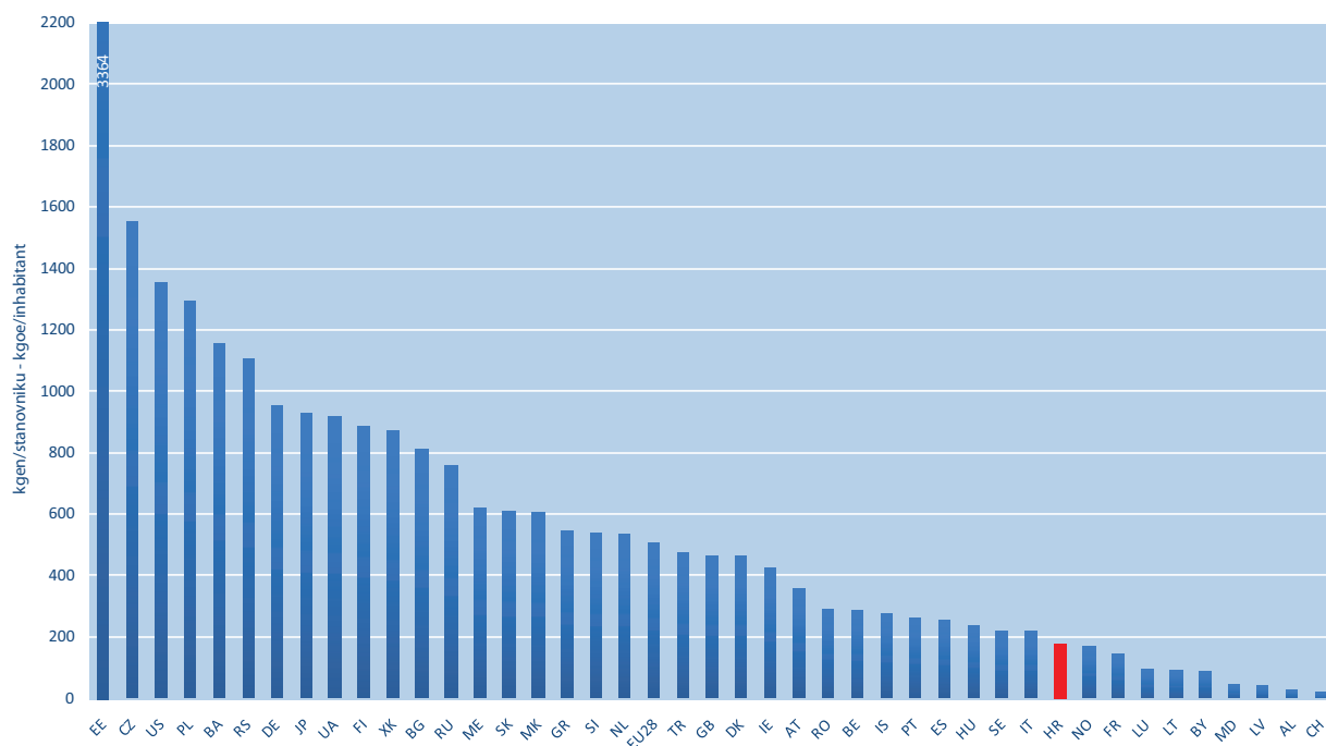
Slika | Figure 2.4.6. Ukupna potrošnja ugljena i koksa po stanovniku | Total consumption of coal and coke per capita Izvor | Source: EIHP
