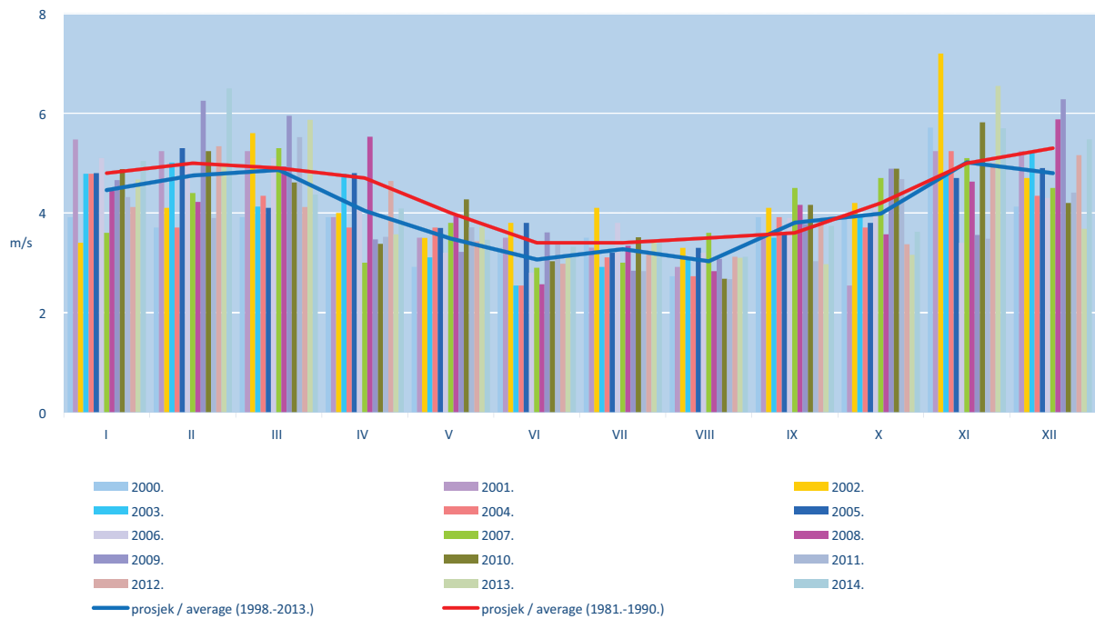
Slika | Figure 8.1.7. Split – Marjan, srednja brzina vjetra | Split – Marjan, Average wind speed Izvor | Source: DHMZ
