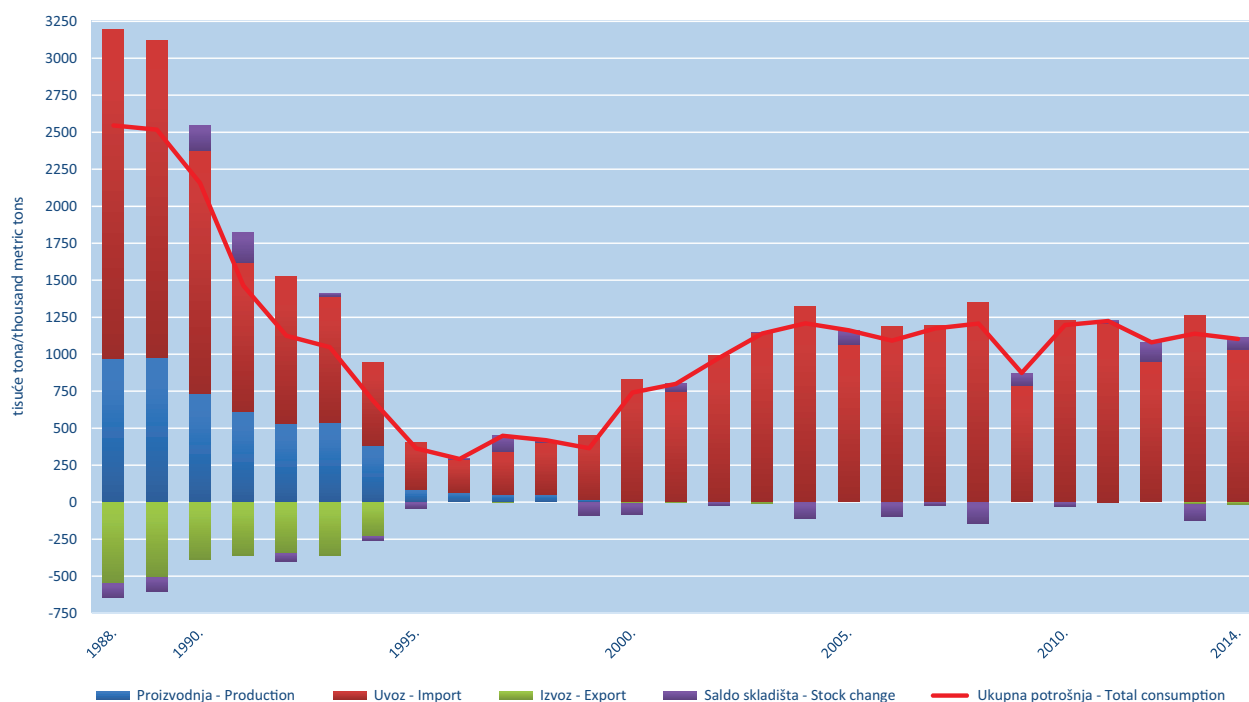
Slika | Figure 7.2.1. Raspoložive količine ugljena i koksa u Hrvatskoj | Coal and Coke Supply in Croatia
