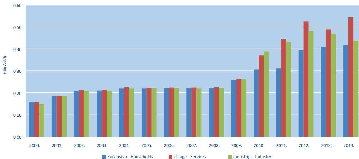
Slika | Figure 4.5.1. Kretanje prosječne prodajne cijene prirodnog plina od 2000. do 2014. godine (s PDV-om) |
