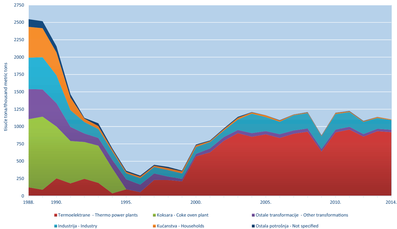
Slika | Figure 7.2.2. Potrošnja ugljena i koksa u Hrvatskoj | Coal and coke consumption in the Republic of Croatia
