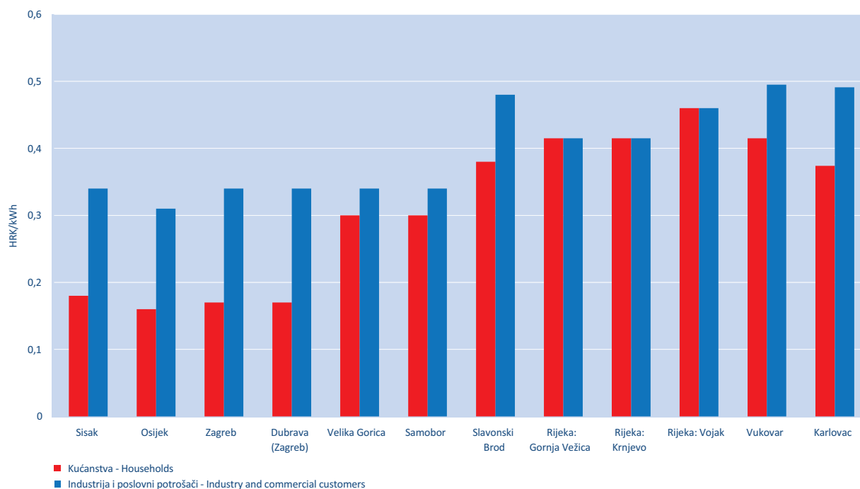
Slika | Figure 6.4.1. Usporedba visina tarifnih stavki centralnih toplinskih sustava pojedinih toplinarskih tvrtki za tarifni element isporučene energije, po kategorijama kupaca (bez PDV-a), na kraju 2014. | Comparison of tariff items (without tax) for energy by customer categories for central DH systems of district heating companies, at the end of 2014 – Izvor | Source: EIHP
