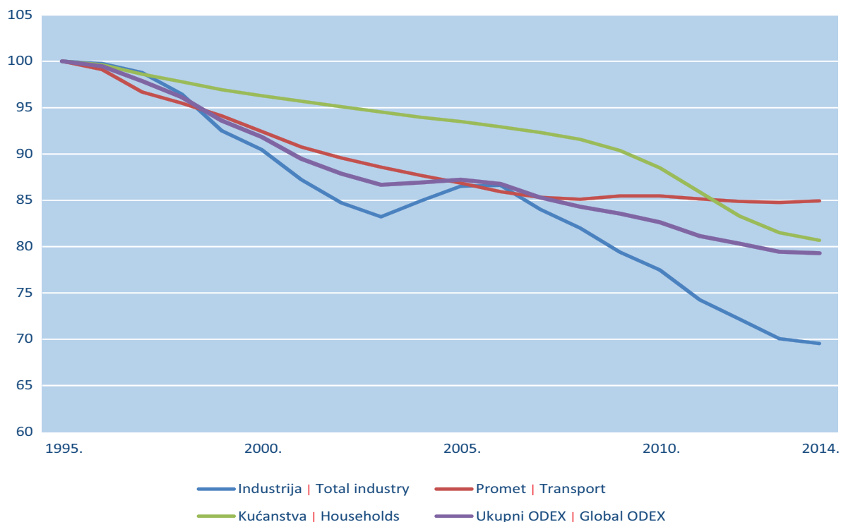
Slika | Figure 9.1.1. Indeks poboljšanja energetske učinkovitosti ODEX | Energy efficiency index ODEX for all sectors - Izvor | Source: EIHP
