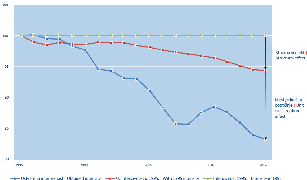
Slika | Figure 9.1.4. Energetska intenzivnost i strukturni makroekonomski efekt za razdoblje od 1995. do 2012. (1995=100) | Energy intensity and structural macroeconomic effect from 1995 to 2012 (1995=100) Izvor | Source: EIHP
